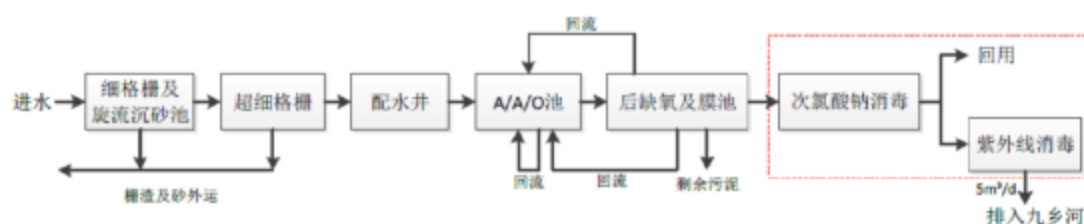
图 4-3 仙林污水处理厂工艺流程图
